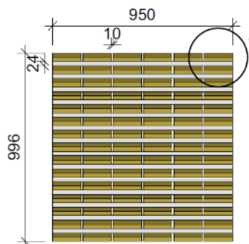
Bretter (3-Seitig sichtbar)
